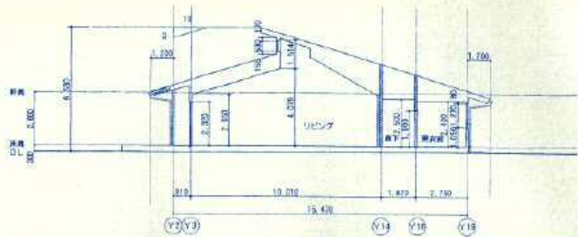
(X1) 断面図 S=1/100
