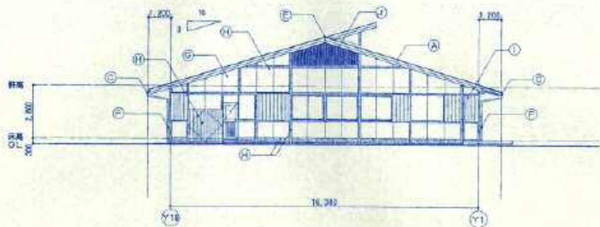
西立面図 S=1/100
