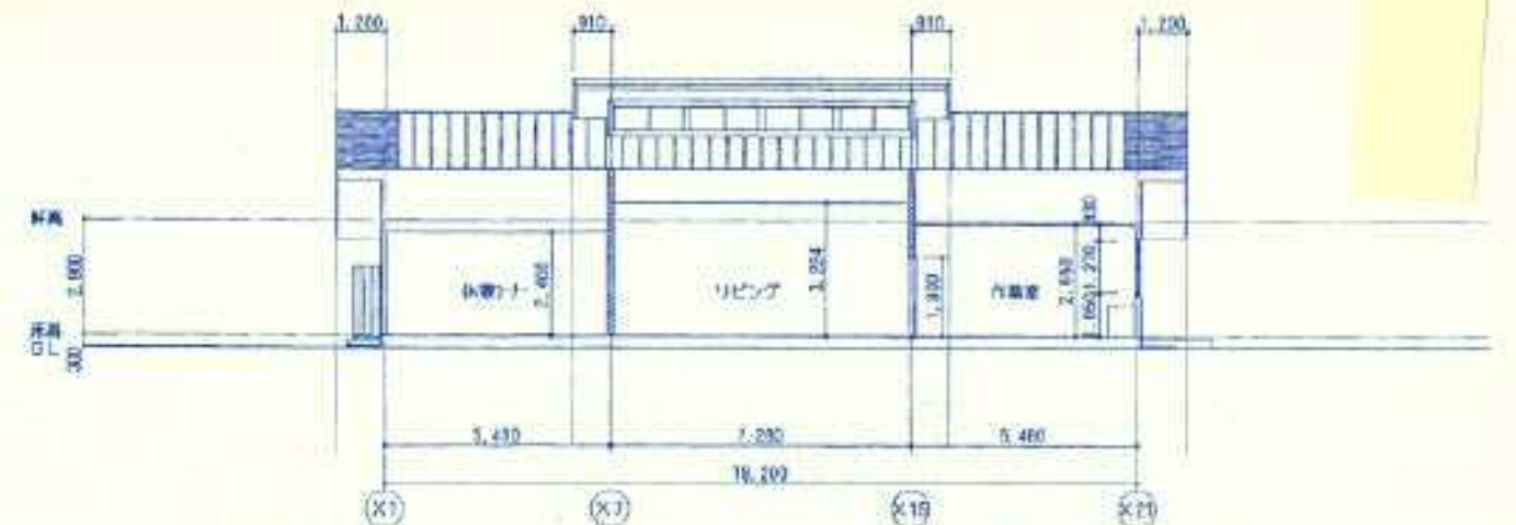
(Y5) 断面図 S=1/100
